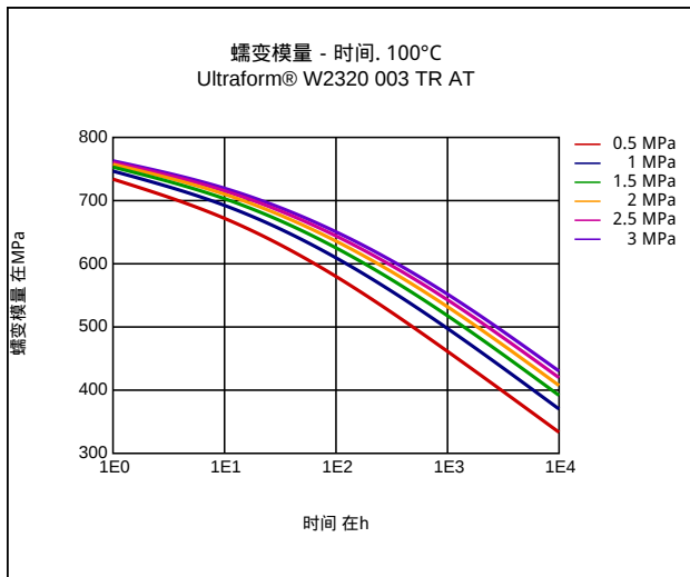
蠕变模量 - 时间, 100°C
